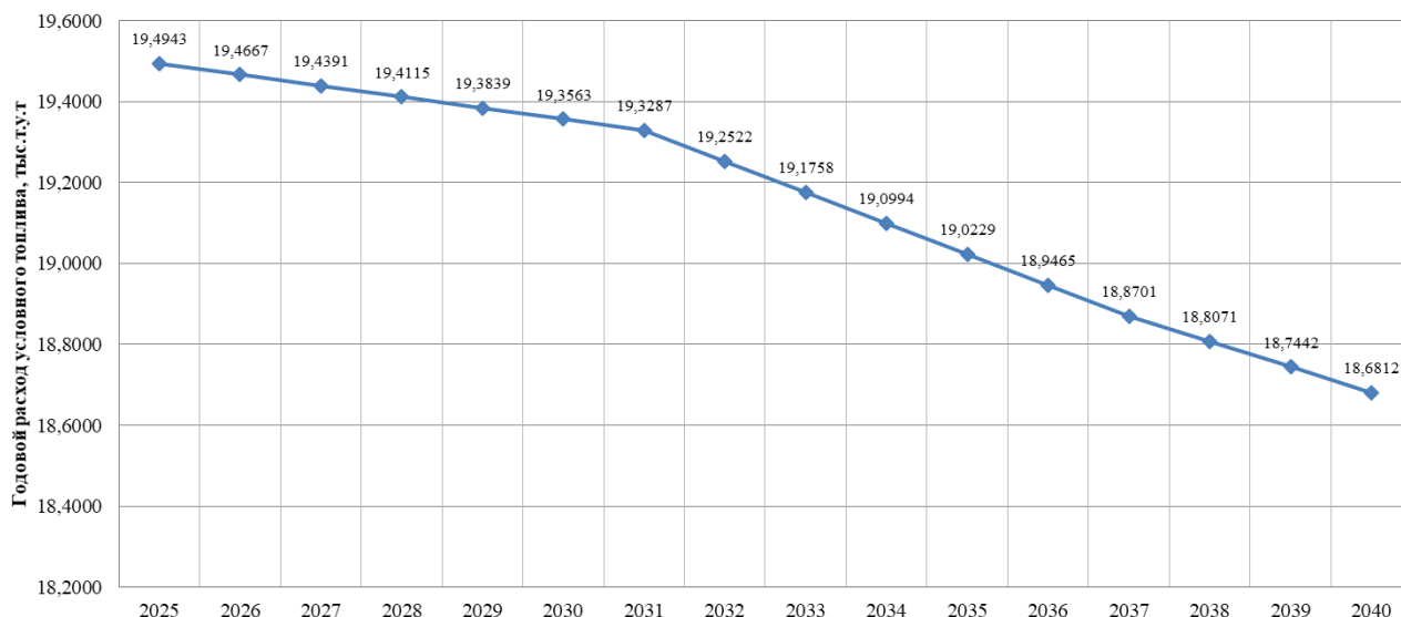
Рисунок 32. Перспективный баланс Тяжинского муниципального округа по твердому топливу
