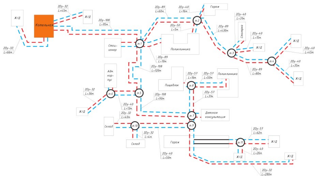
Рисунок 16. Границы зоны ЦСТ - «Итатская больница»
