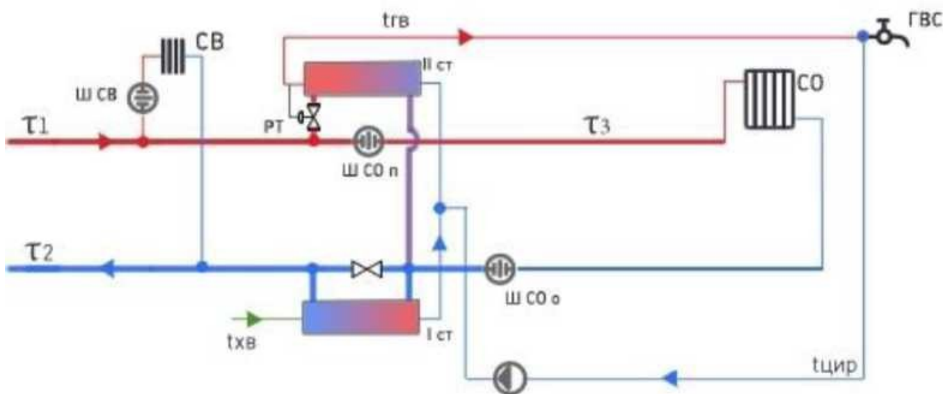
Рисунок 30. Двухступенчатая (смешенная) схема присоединения подогревателей ГВС с зависимым присоединением системы отопления
