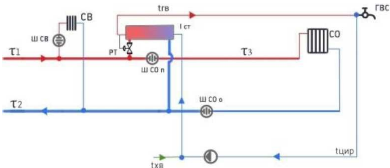
Рисунок 29. Одноступенчатая (параллельная) схема присоединения подогревателей ГВС с зависимым присоединением системы отопления
