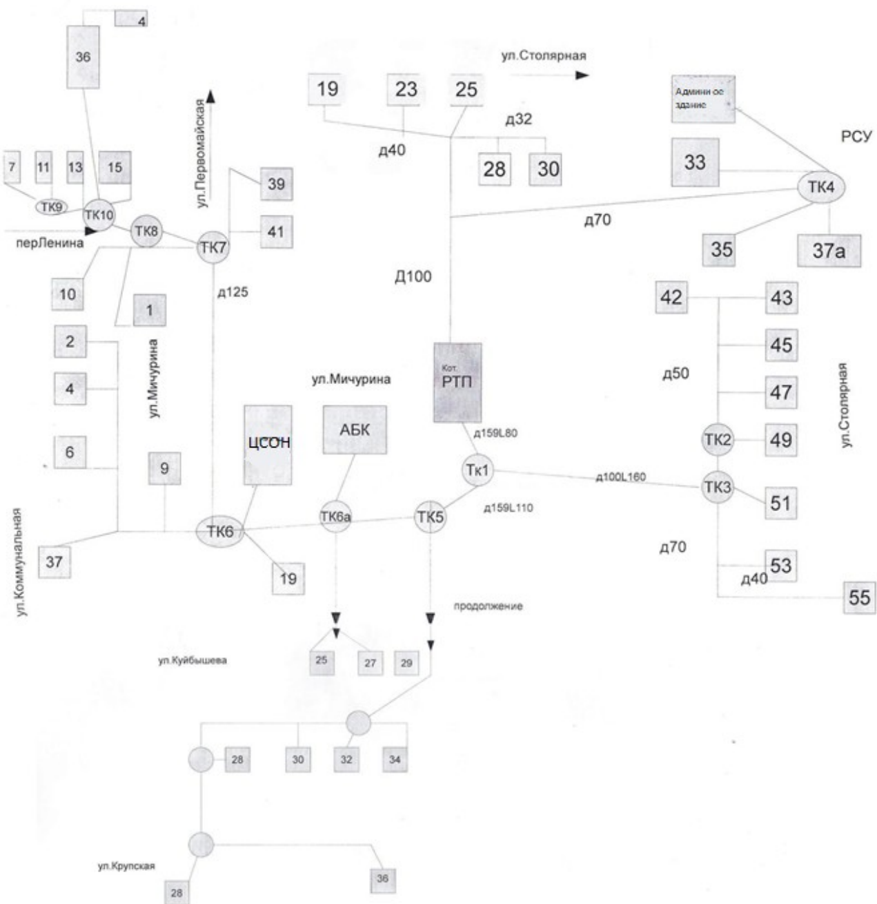
Рисунок 8. Границы зоны ЦСТ - «РТП»
