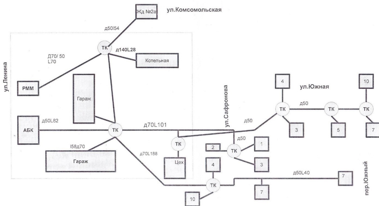
Рисунок 28. Границы зоны ЦСТ - «ЗАО Тяжинское ДРСУ»
