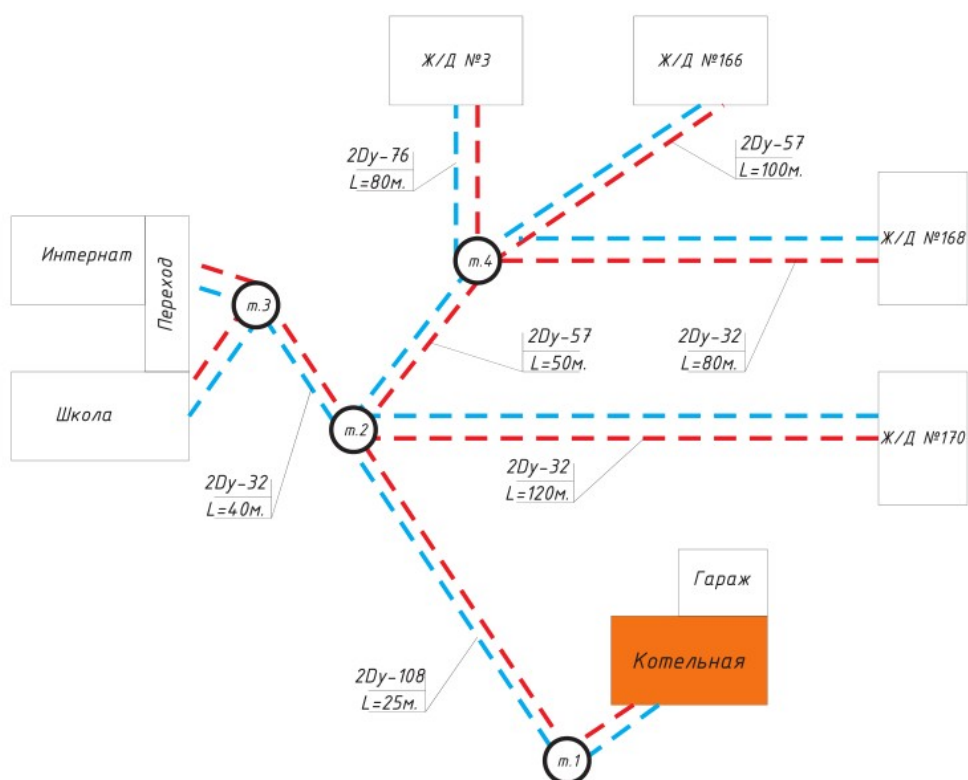
Рисунок 15. Границы зоны ЦСТ - «Итатская ср. школа»
